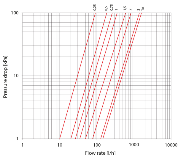
График клапана, регулирующего расход (коллектор подачи)
