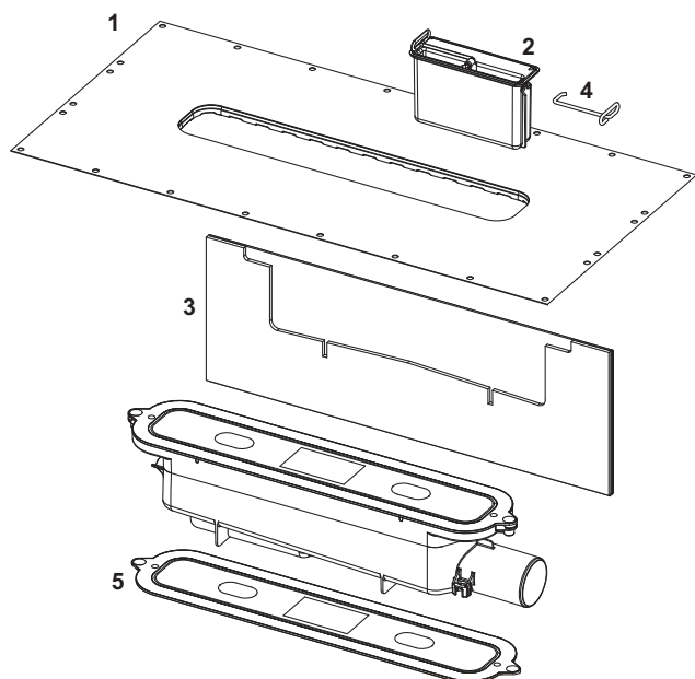
Сифон TECEdrainprofile, стандартний, з горизонтальним відводом DN 50
