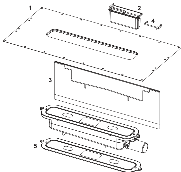
Сифон TECEdrainprofile, «flat», з горизонтальним відводом DN 40
